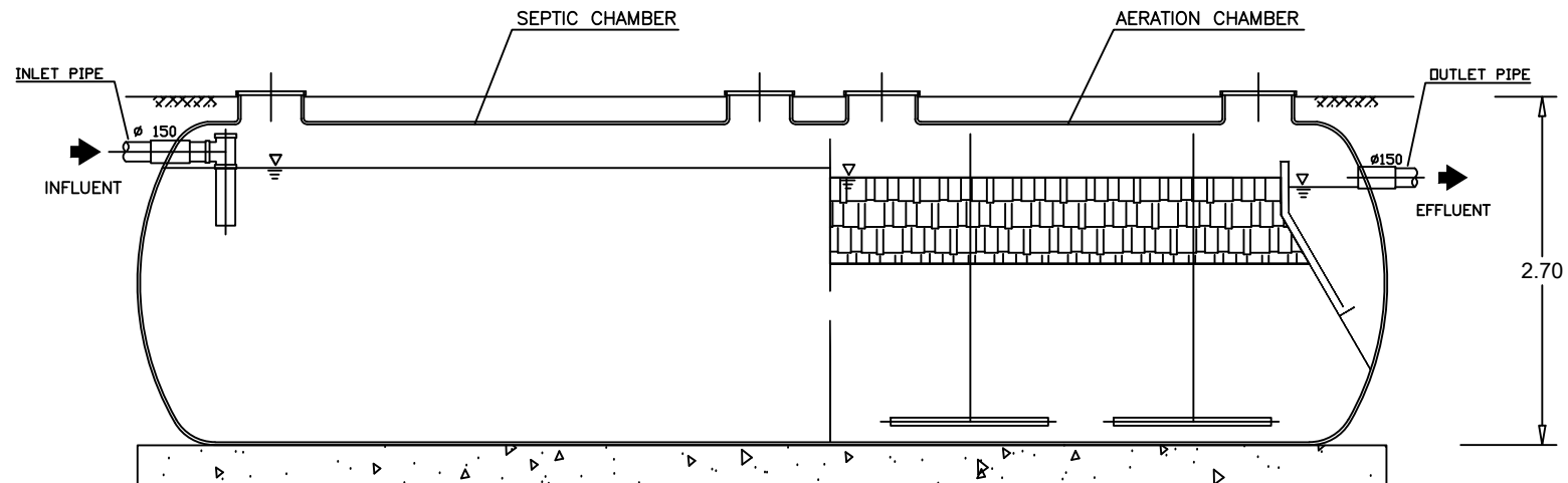
SECTION A-A
