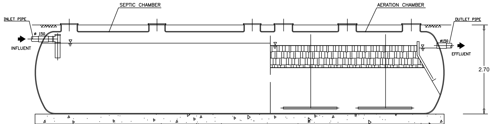
SECTION A-A
