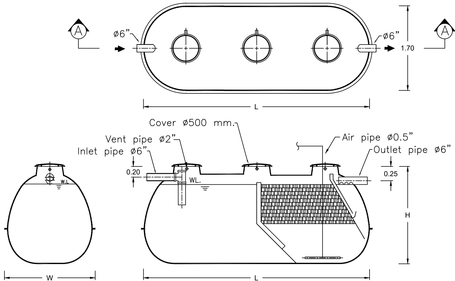
SECTION A-A
