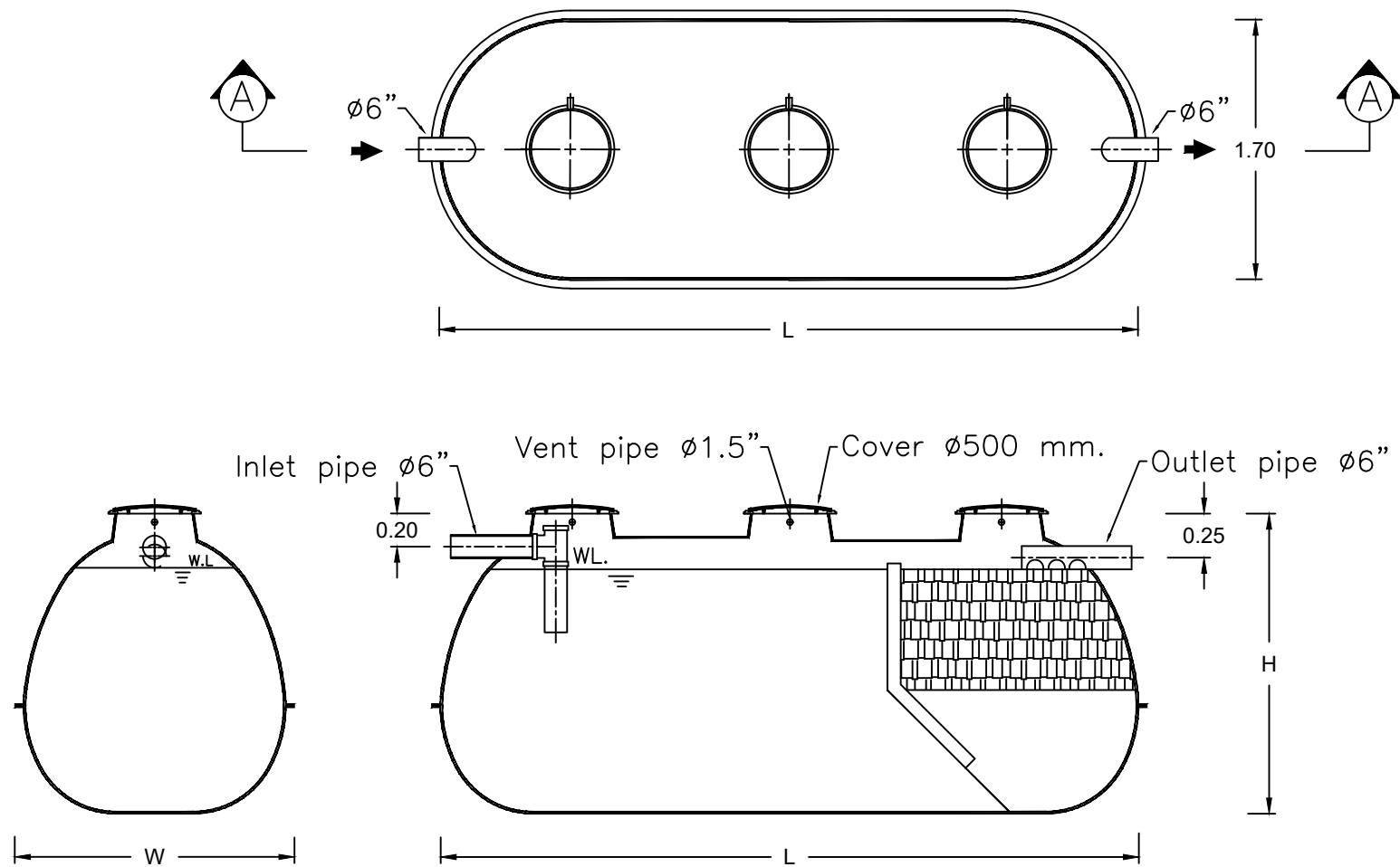
SECTION A-A
